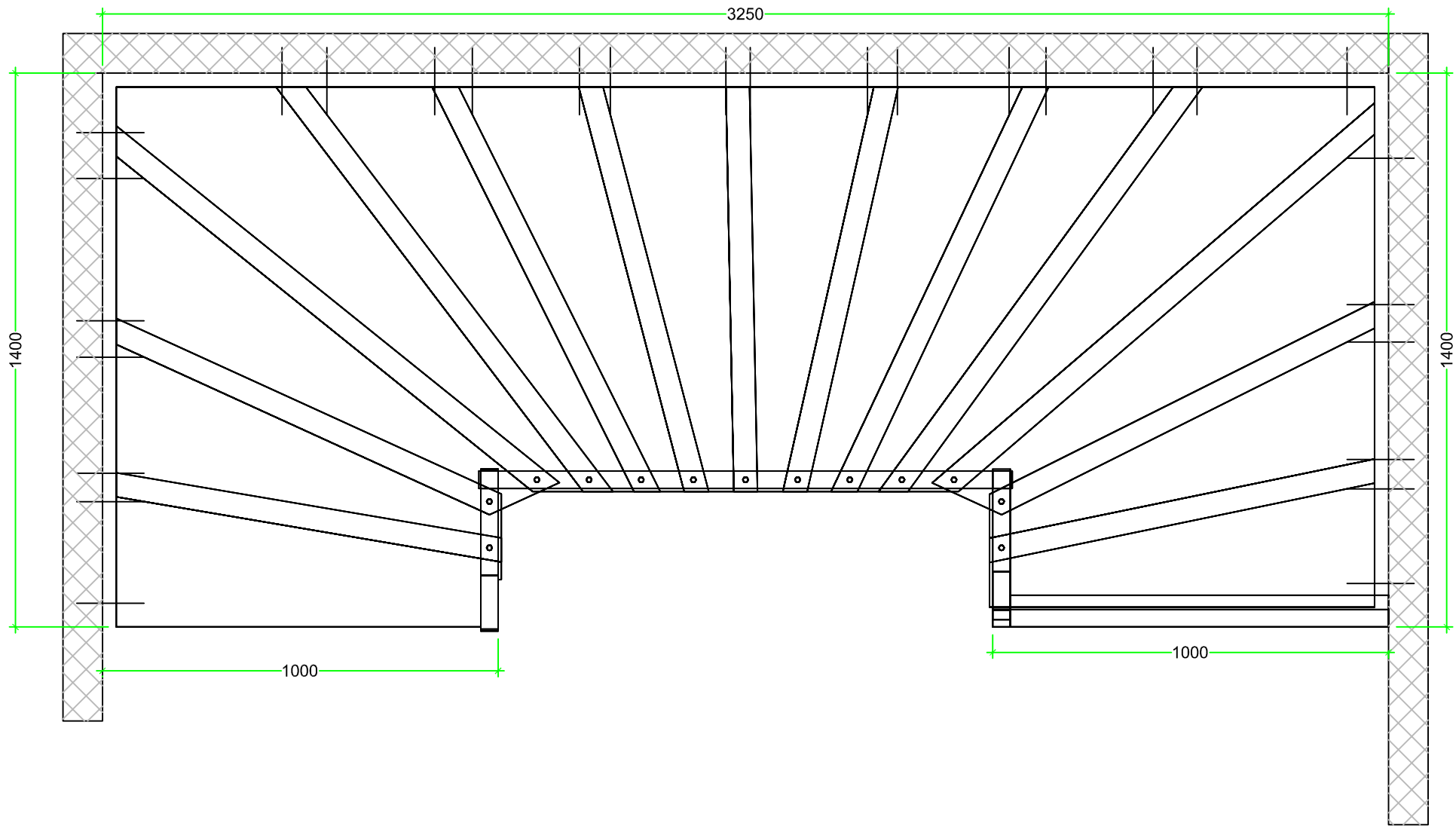
Halbgewendelte Treppe
