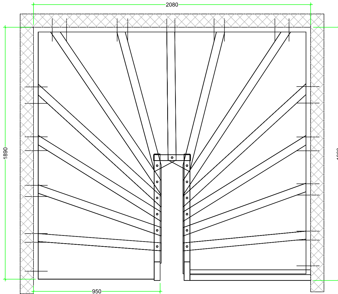
Halbgewendelte Treppe
